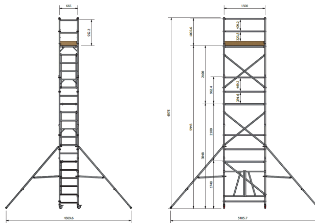
Bild 1: Gesamtübersicht Typ Eurofold 1,5 x 0,6 m; Maße in [mm]
