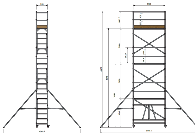
Bild 2: Gesamtübersicht Typ Eurofold 1,9 x 0,6 m; Maße in [mm]
